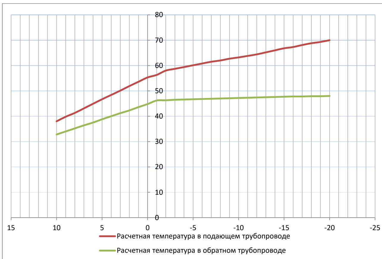
Рисунок 5.1 – Температурный график тепловых сетей
