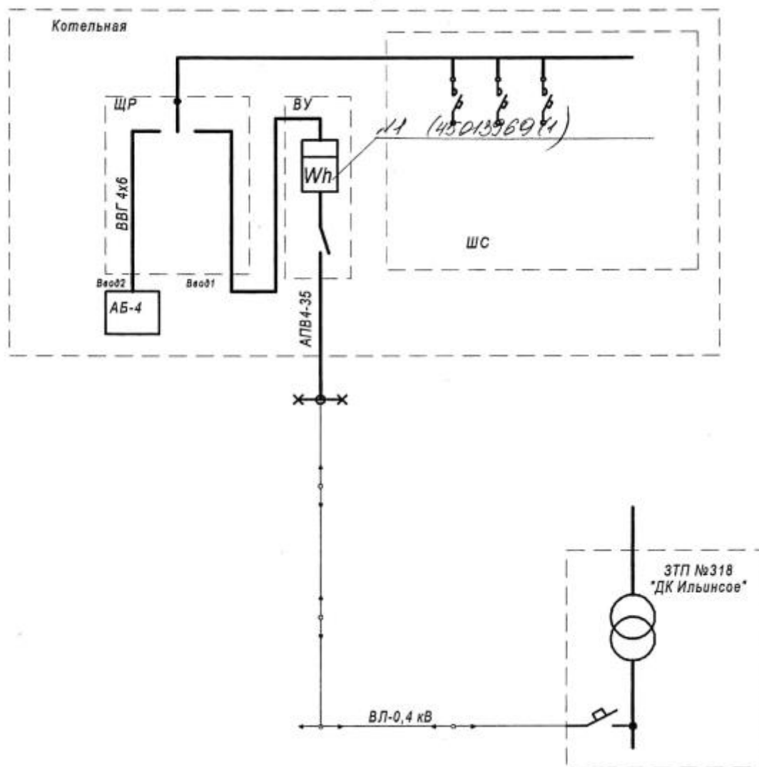
Рисунок 1.2.1 – Схема электроснабжения центральной котельной
