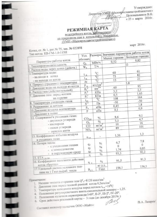
Рисунок 1.2.4 – Режимная карта котла 1 центральной котельной
