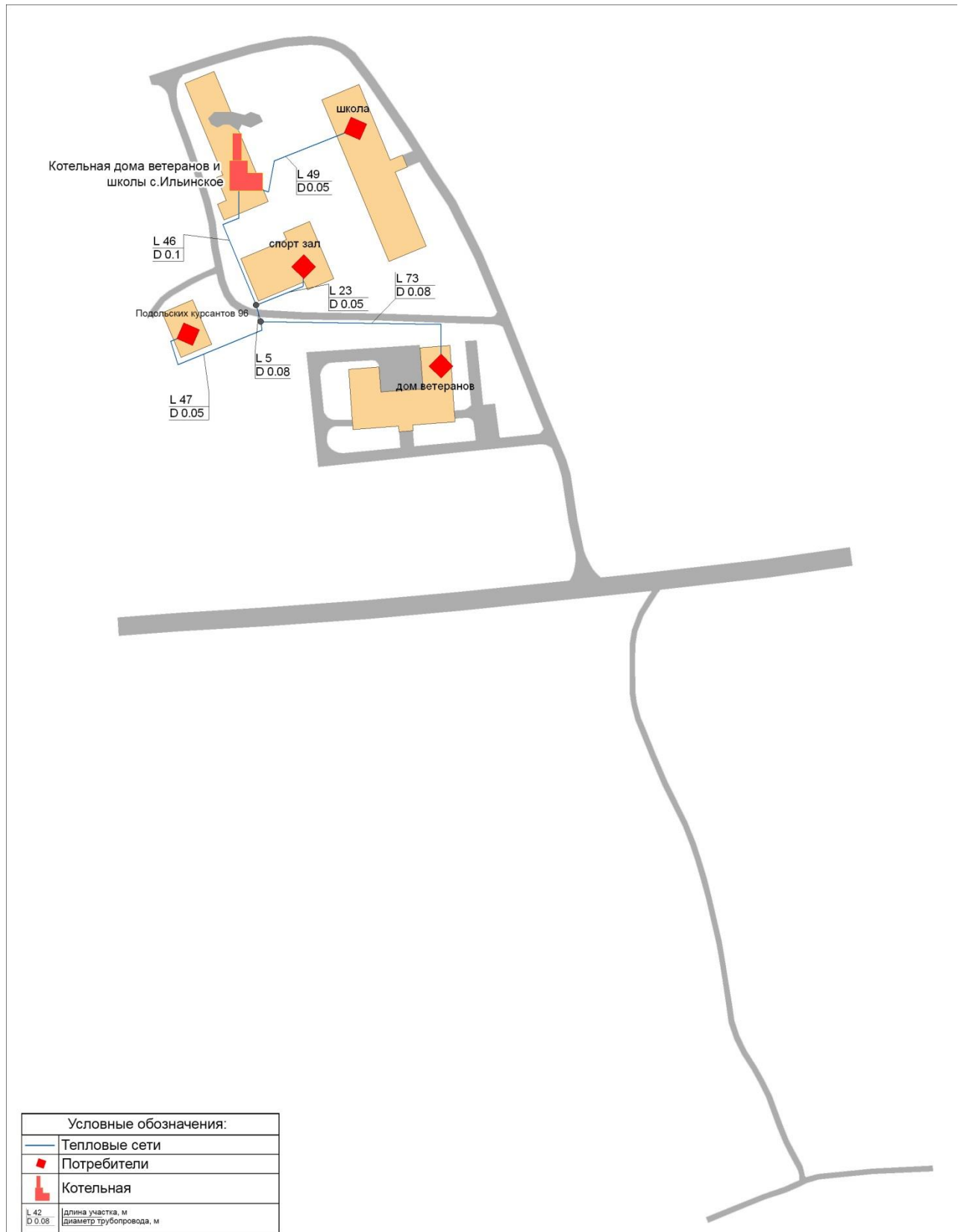
Рисунок 1.3.2 – Схема тепловых сетей котельной дома ветеранов и школы с. Ильинское
